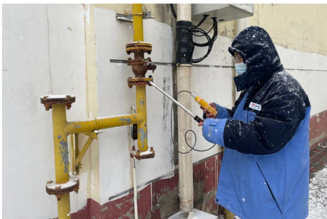
蓟州公司巡维抢人员王冉对户外管网及调压设备进行检测
